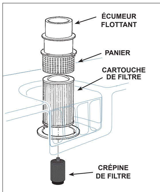
SYSTÈME DE FILTRE
