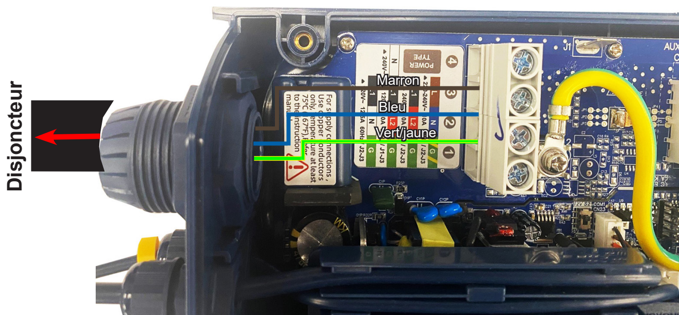
Boîtier de commande
